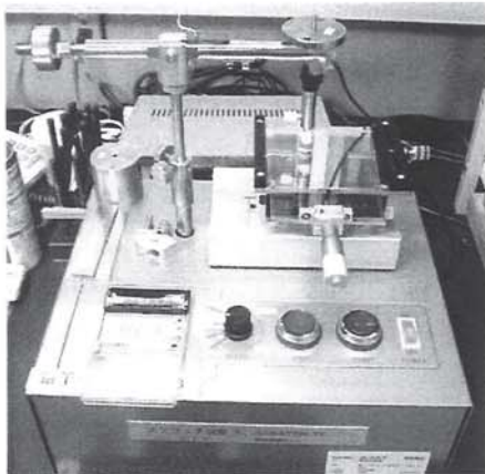
写真1 スクラッチ試験機
